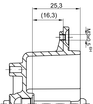
Corte A-A
