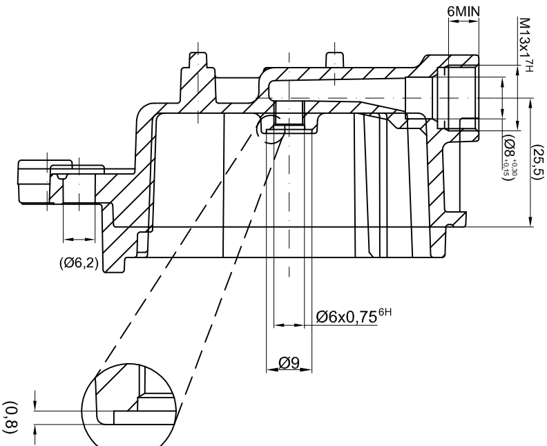
Corte B-B
